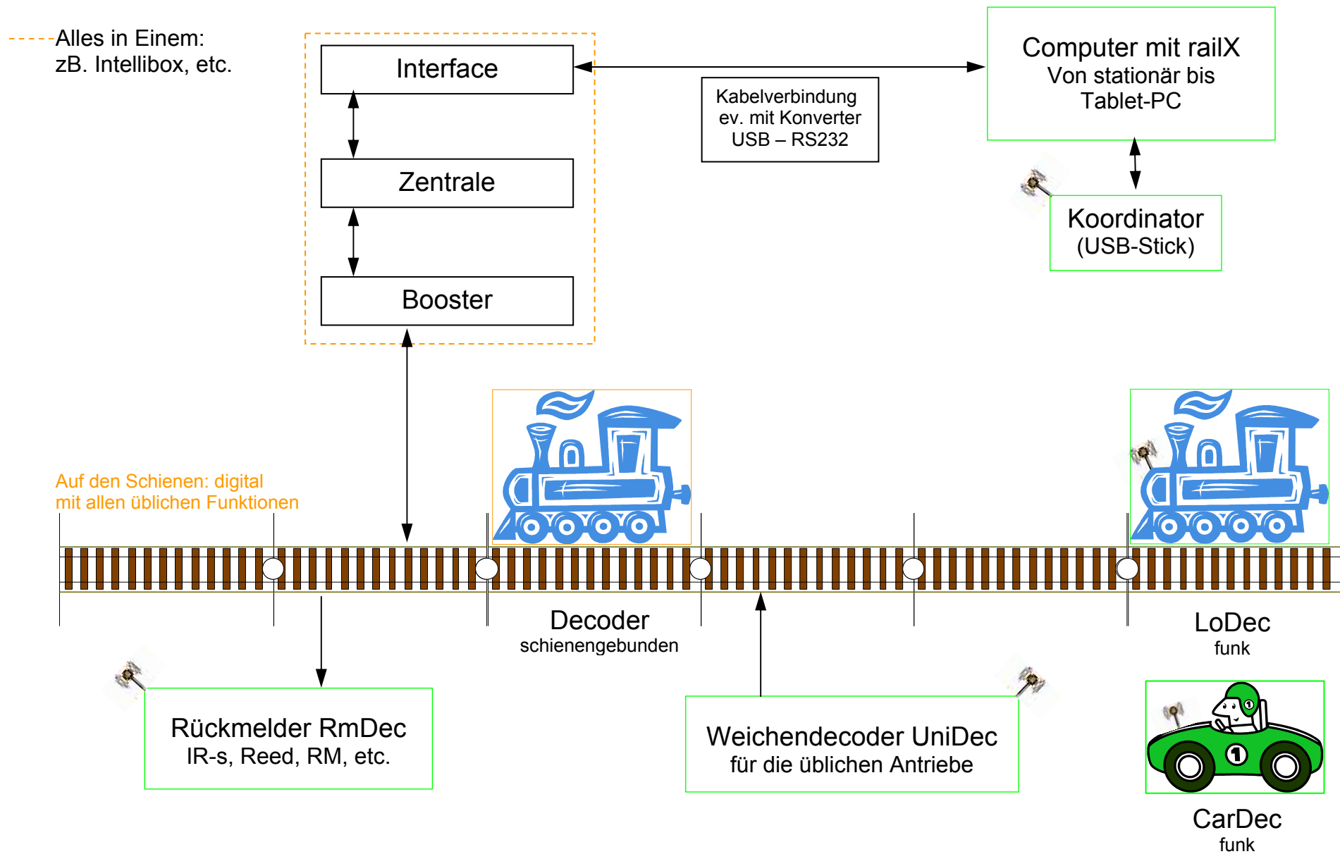
Fig. 3) Komponenten „RailCommander“ kompatibel mit Digitalsteuerung
